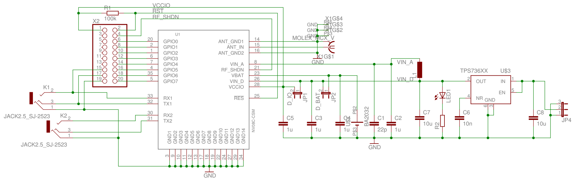
sysmocom NVS GPS evaluation module v3
